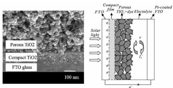
图2 具有 \text{TiO}_2 密集层的 SEM 截面图 及其 DSC 结构示意图
