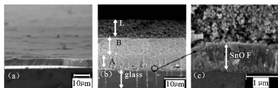
(a)小颗粒致密层,(b)光阳极整体结构, (c) \text{TiO}_2 层和导电玻璃交界处
